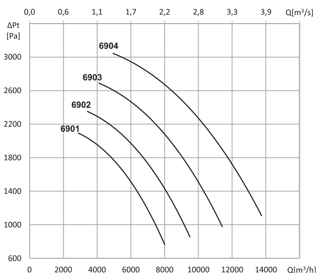
Charakterystyki przepływowe:
